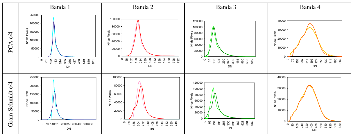
Figura 3: Histogramas comparativos das fusões Principais componentes e Gram-Schmidt . As linhas com cores mais claras representam os histogramas das imagens originais e as linhas mais escuras representam os histogramas das imagens sintéticas simuladas.
